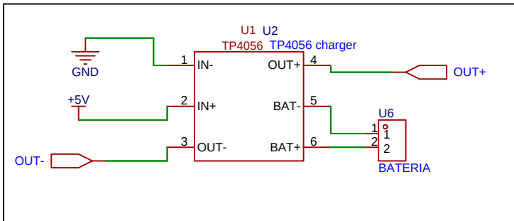
MODULO TP4056
