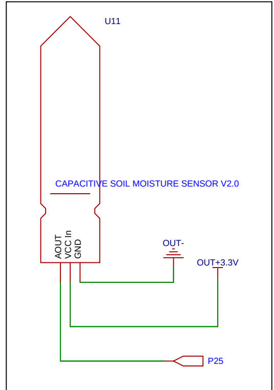
SENSOR HUMEDAD ANALOG
